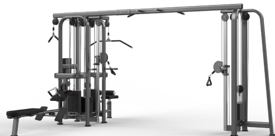
FM-1006 6-STATIONEN-TURM
